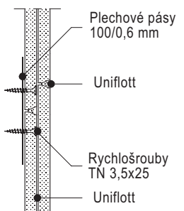
Dvouvrstvý - slepený čelní hrany předsazené
